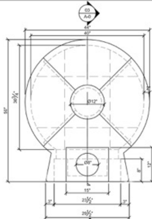
01 OVEN PLAN A-0 SCALE: 3/4"=1'-0"
