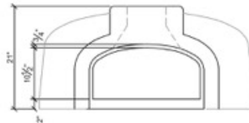
02 FRONT ELEVATION A-0 SCALE: 3/4"=1'-0"
