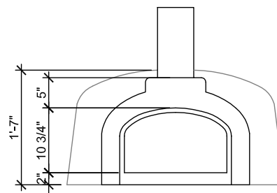
02 FRONT ELEVATION A-1 SCALE: 3/4"=1'-0"
