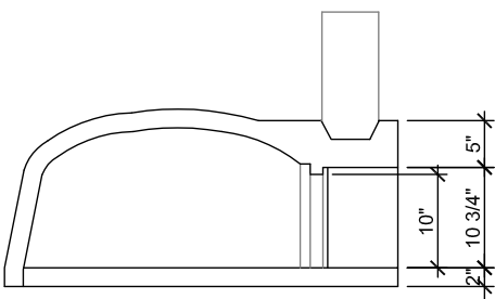
03 SIDE ELEVATION A-1 SCALE: 3/4"=1'-0"
