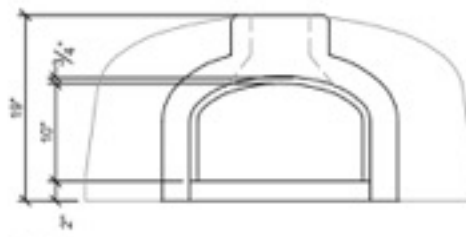
02 FRONT ELEVATION A-0 SCALE: 3/4"=1'-0"
