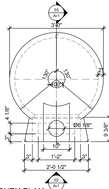
01 OVEN PLAN A-1 SCALE: 3/4"=1'-0"
