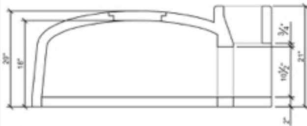
03 SIDE ELEVATION A-0 SCALE: 3/4"=1'-0"
